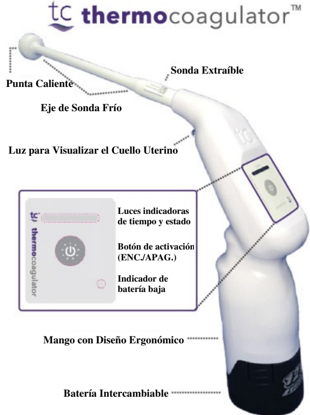
Figura 1: Diseño de tc thermo coagulator™
